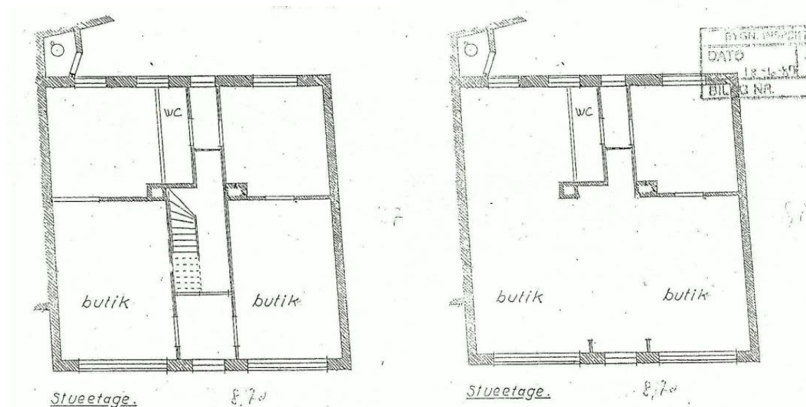
Etageplan over stueetagen fra 1987 før (til venstre) og efter (til højre) butikssammenlægning. 341
